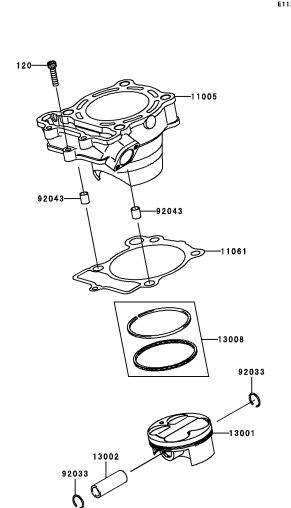
B-5 Cylinder/Piston(s)
