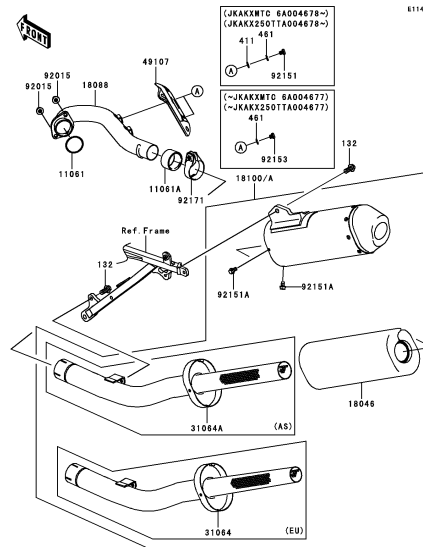
B-7 Muffler(s)
