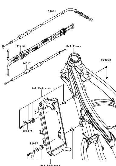
F-13 Cables
