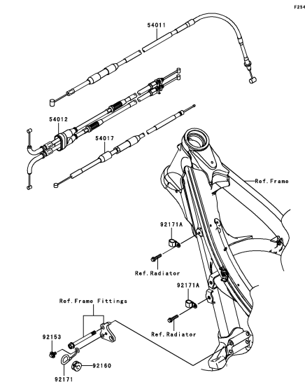
F-14 Cables
