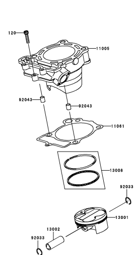
B-5 Cylinder/Piston(s)
