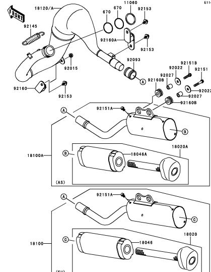
B-5 Muffler(s)
