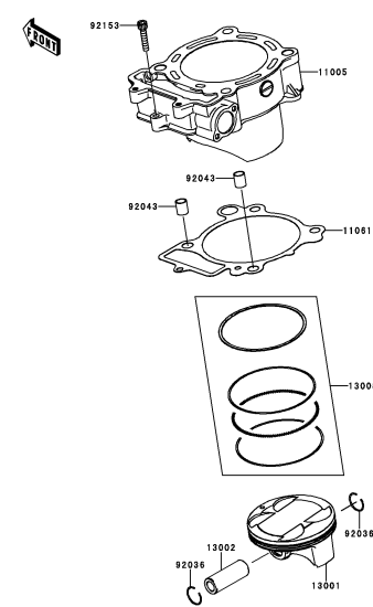
B-5 Cylinder/Piston(s)
