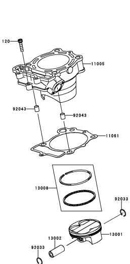
B-5 Cylinder/Piston(s)
