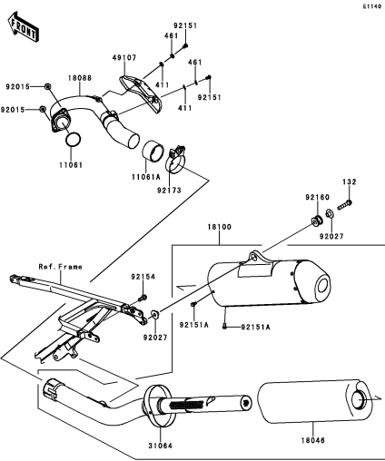
B-7 Muffler(s)
