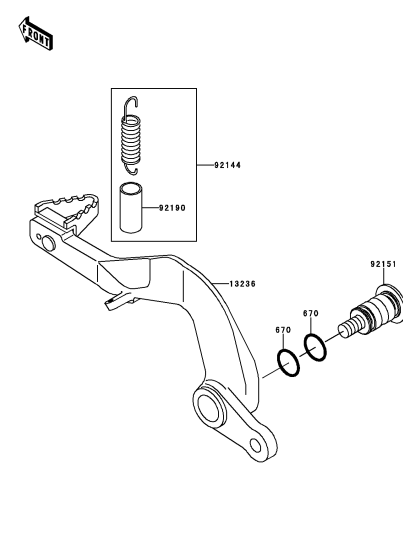
D-14 Brake Pedal
