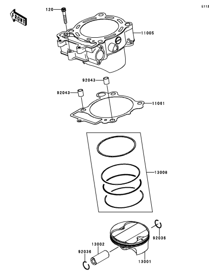
B-5 Cylinder/Piston(s)
