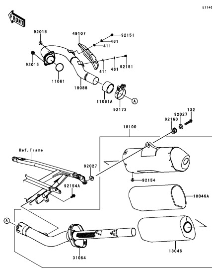
B-7 Muffler(s)
