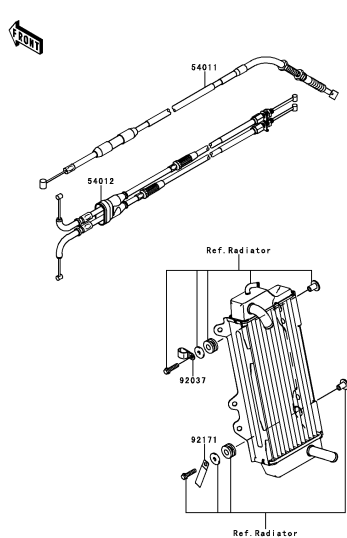
F-12 Cables
