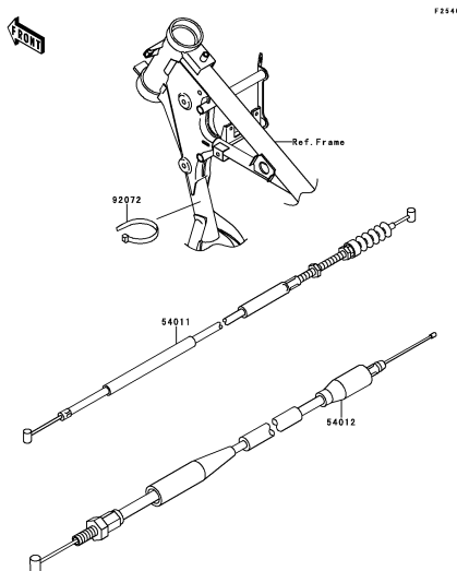
E-12 Cables
