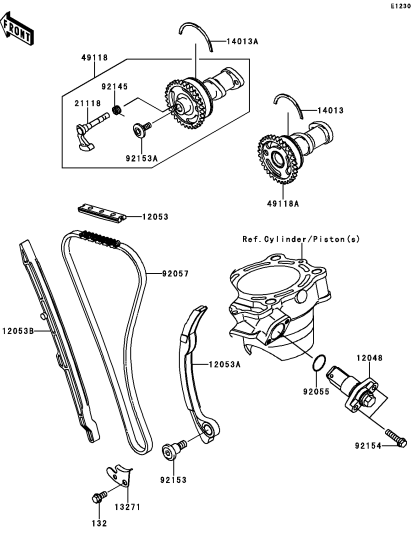
B-10 Camshaft(s)/Tensioner
