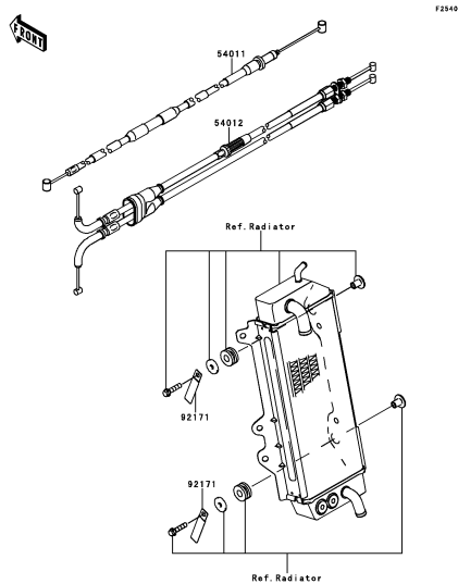
E-12 Cables
