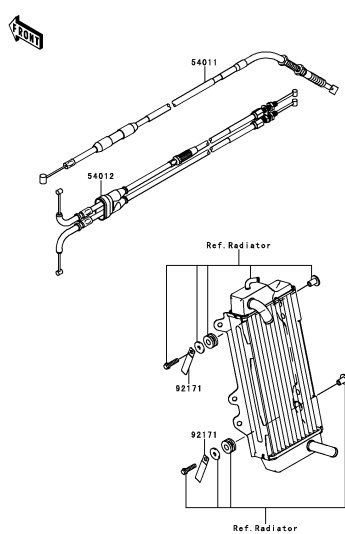
F-12 Cables
