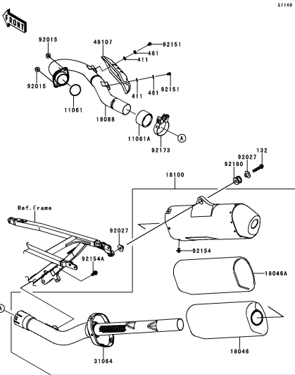
B-7 Muffler(s)
