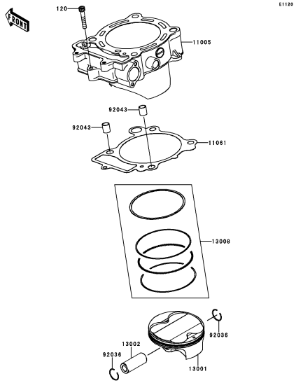
B-5 Cylinder/Piston(s)
