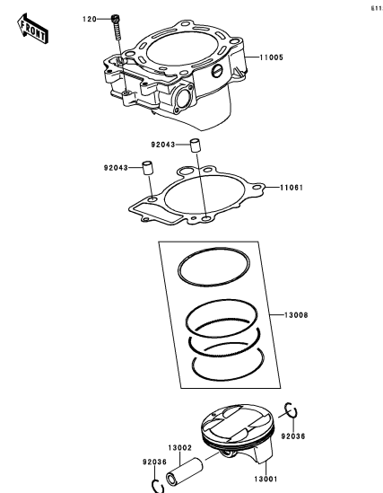
B-5 Cylinder/Piston(s)
