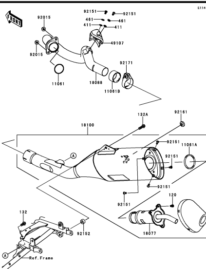
B-7 Muffler(s)
