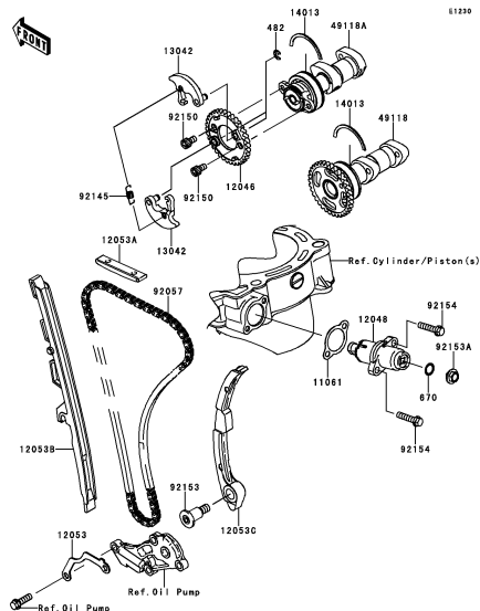
B-9 Camshaft(s)/Tensioner
