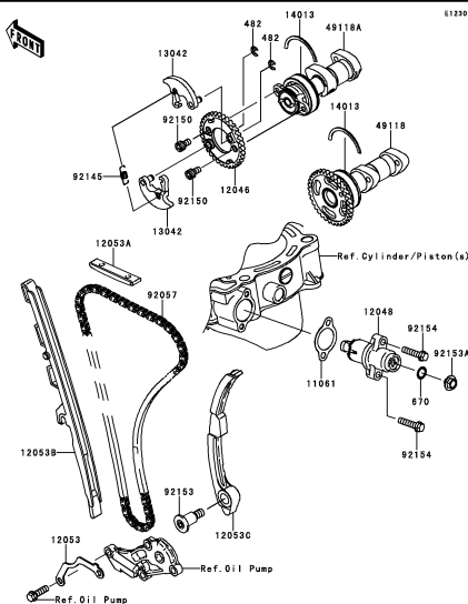
B-9 Camshaft(s)/Tensioner
