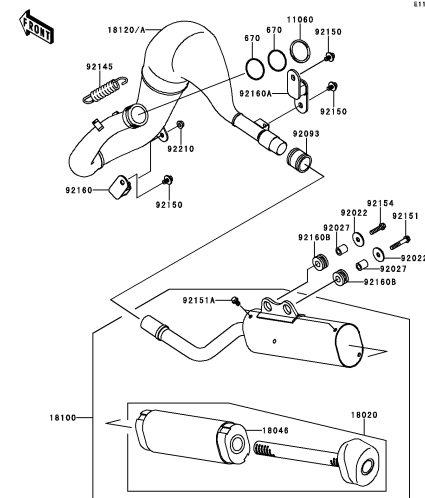
B-5 Muffler(s)
