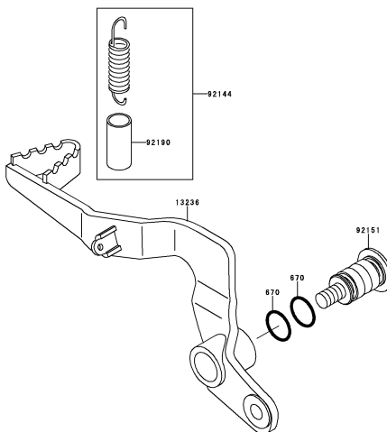
D-13 Brake Pedal
