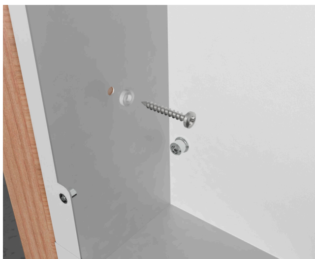
Infästning av skåp i regelvägg
