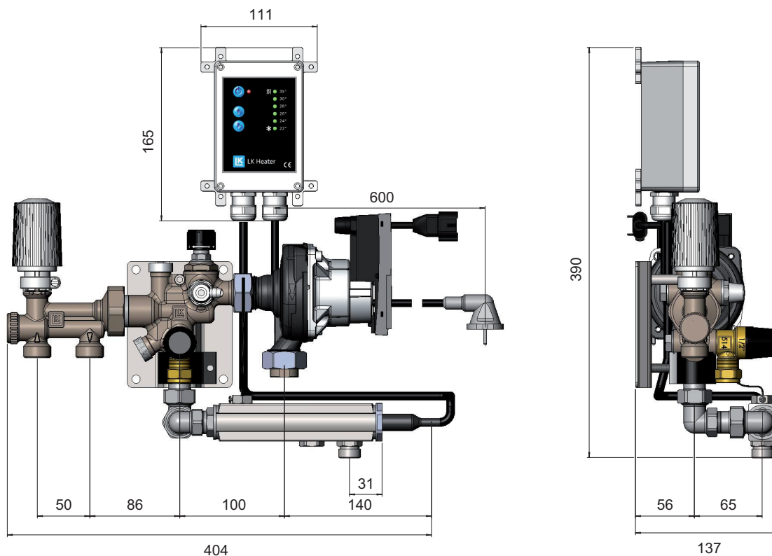
LK Heater för en golvvärme krets monterad med LK Minishunt M60.
