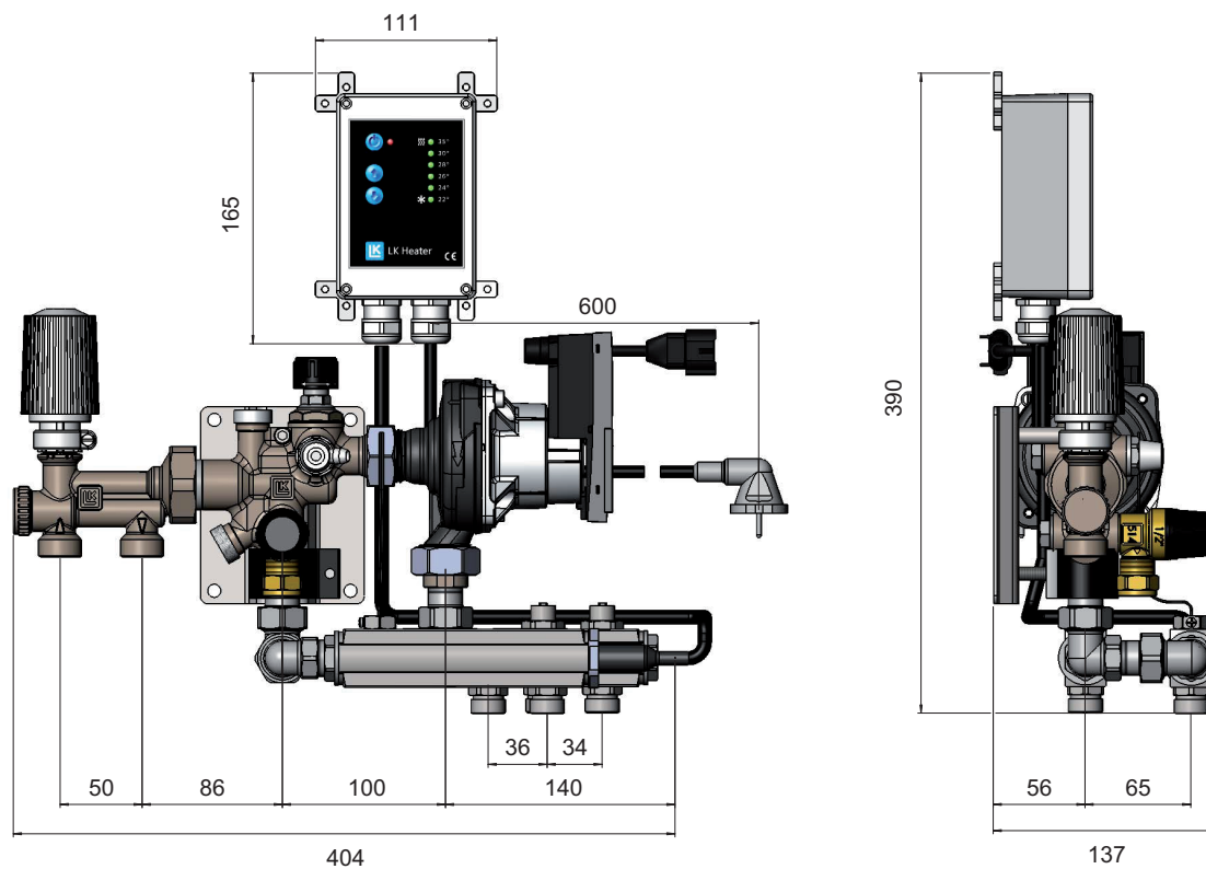
LK Heater för två golvvärme kretsar monterad med LK Minishunt M60.
