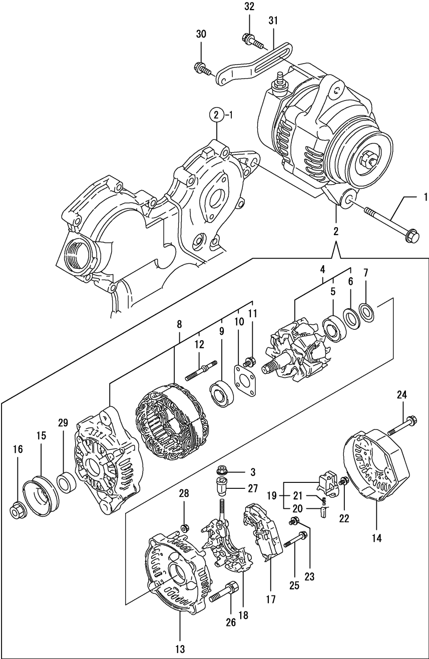
Fig.16. GENERATOR
