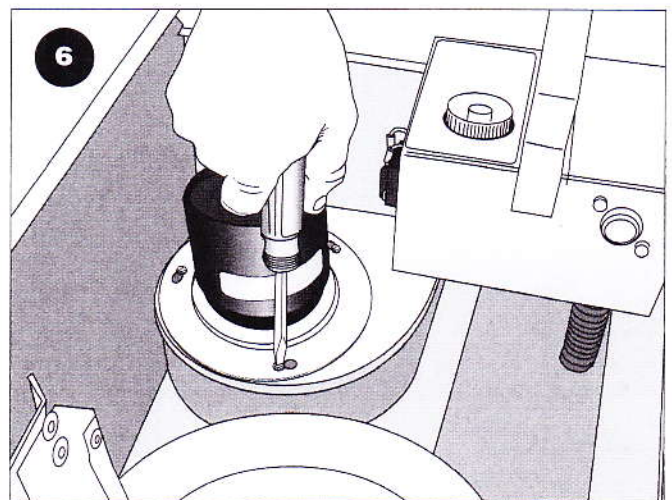
6 Motorn lossas från fästena (3 skruvar) Fortsättning på nästa sida.
