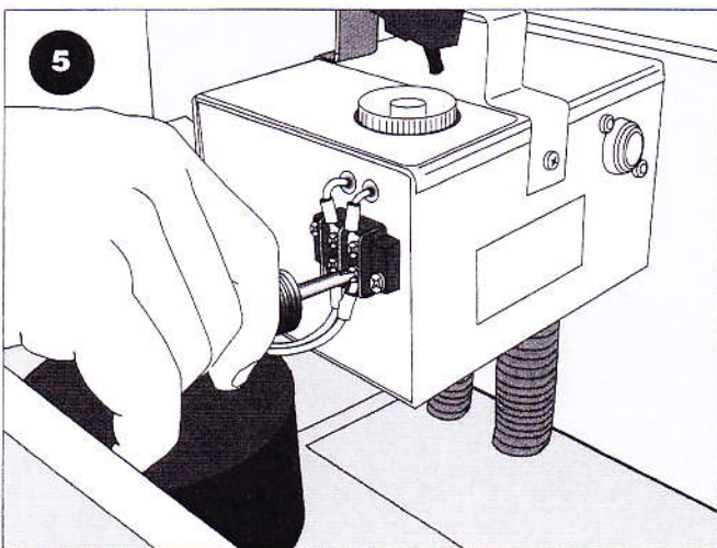
5 Ledningarna till fläktmotorn lossas från kopplingsdosan.
