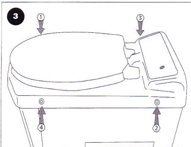
3 Toalettoppen lossas (4 skruvar) se ordningsföljd!
