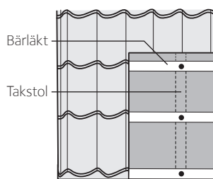
Underlagstak av plastfolie eller board
