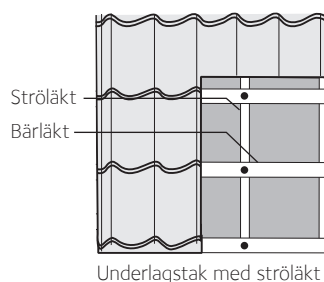
Underlagstak med ströläkt
